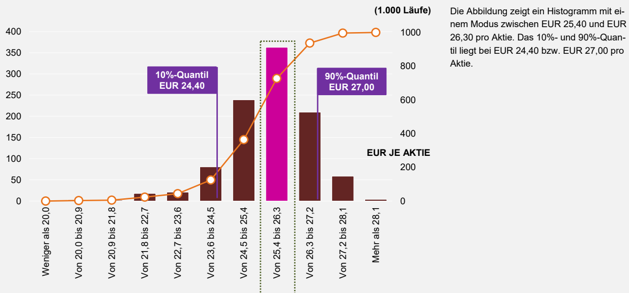
ABBILDUNG 2: MONTE-CARLO-SIMULATION
